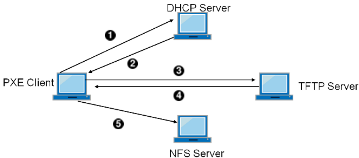
Abbildung 60. PXE-Bootvorgang mit NFS Root Mount
