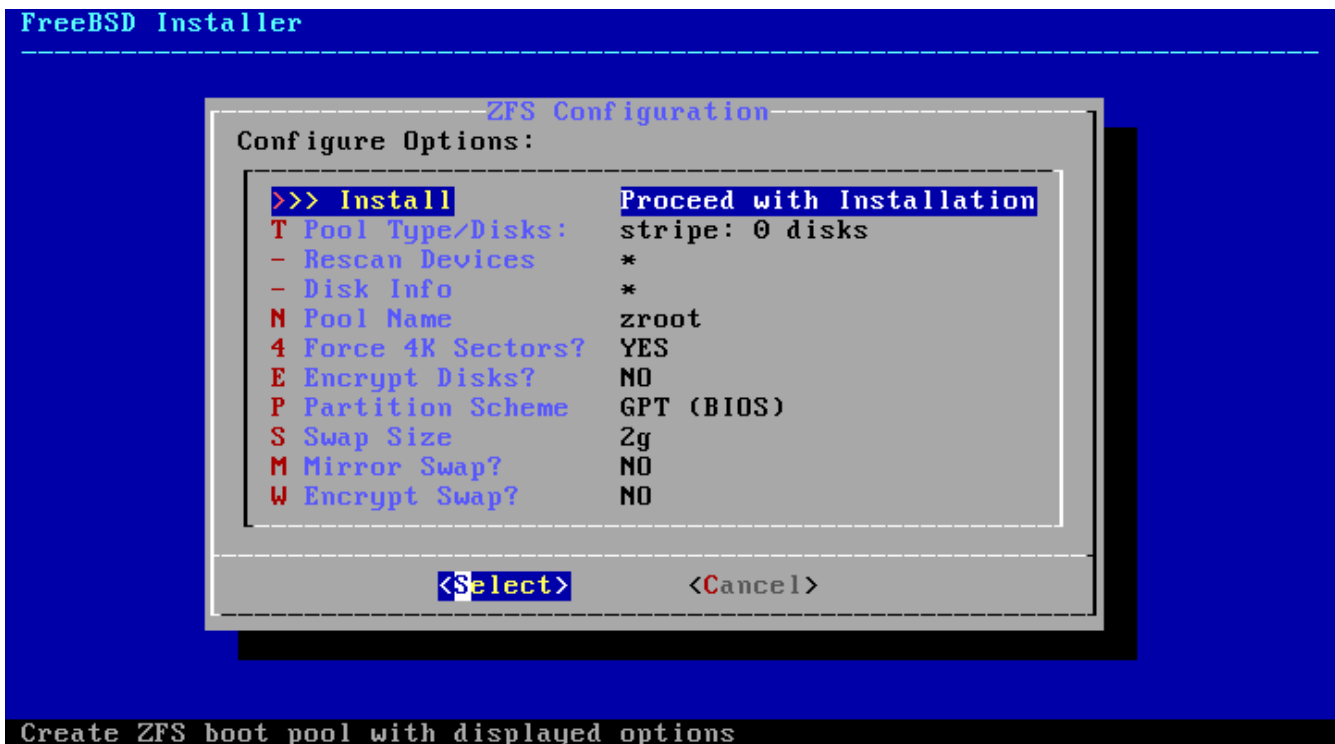
Abbildung 19. ZFS Konfigurationsmenü
