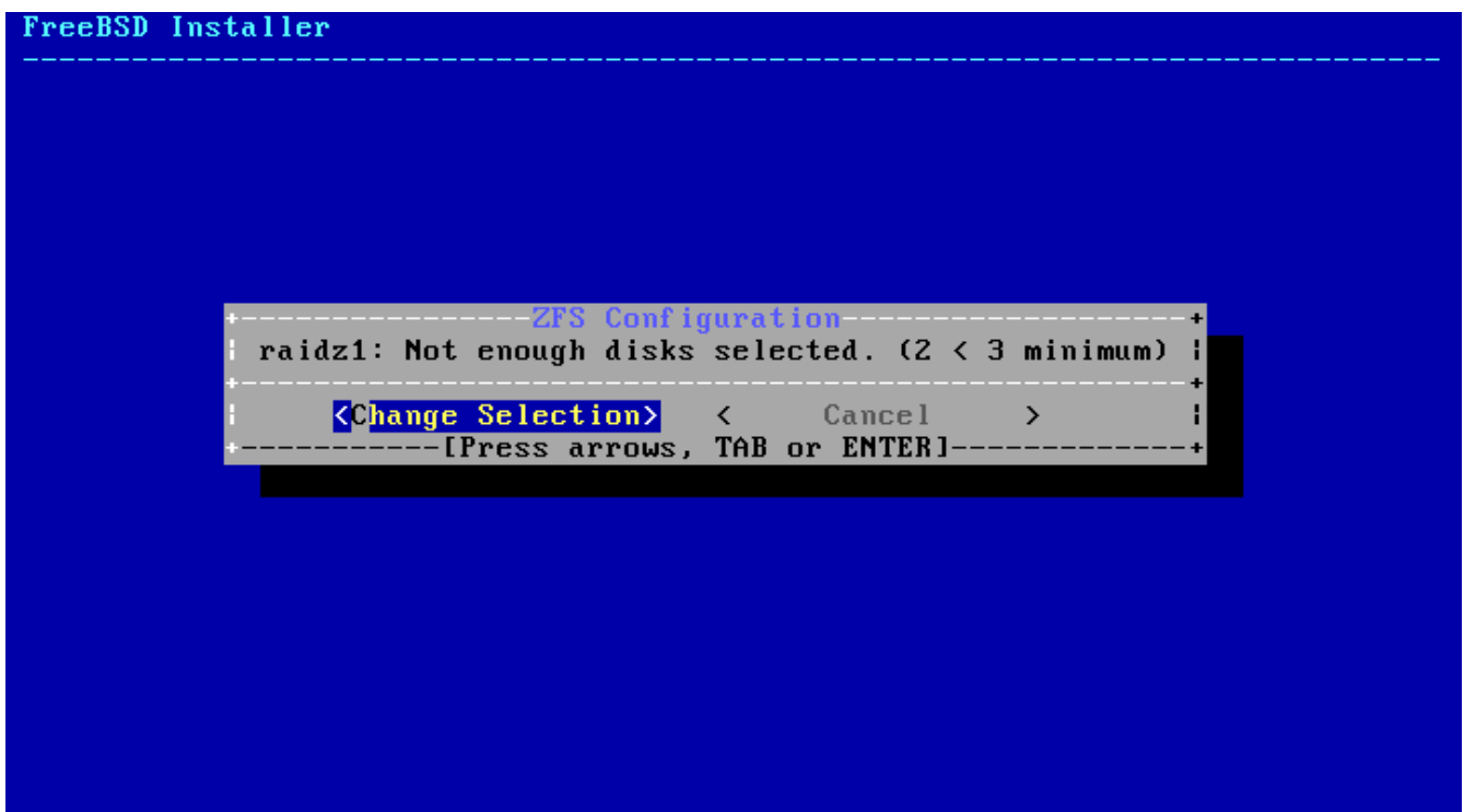
Abbildung 22. Ungültige Auswahl
