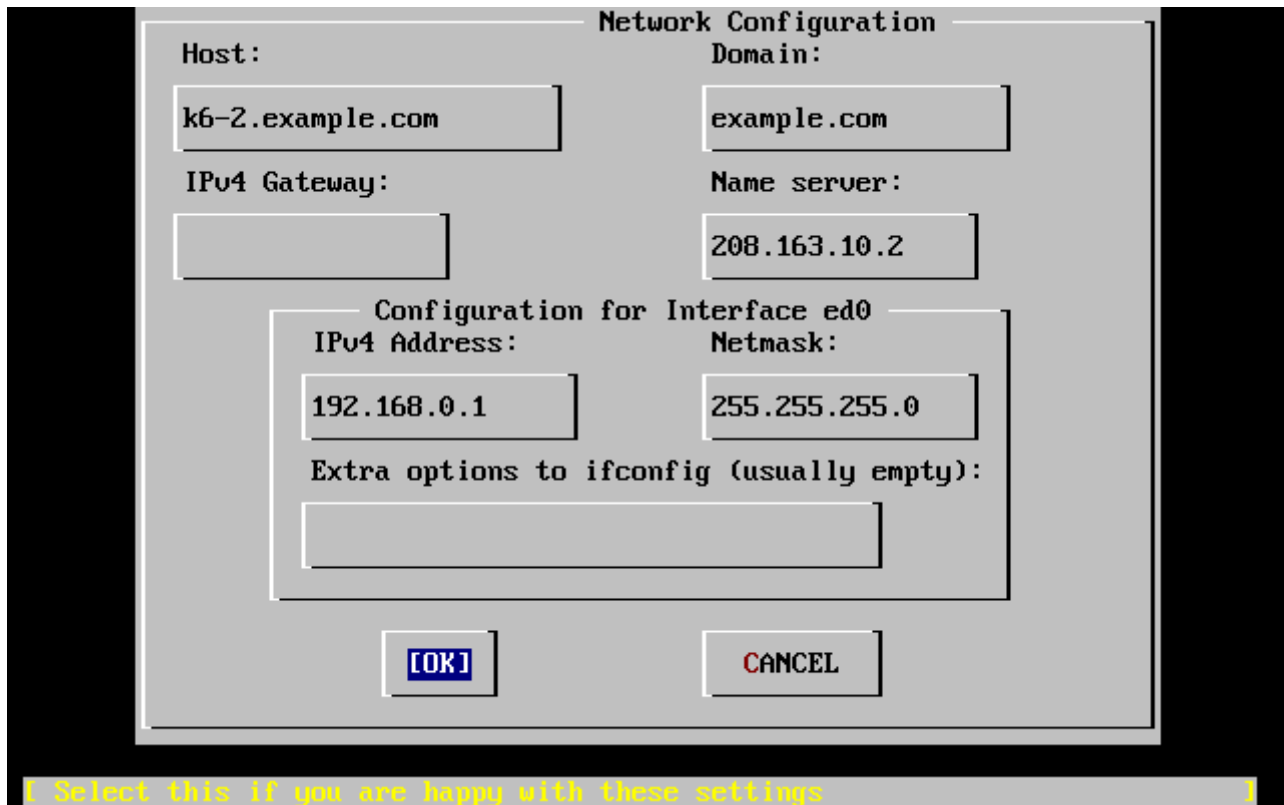
Figuur 28. Netwerkinstellingen voor ed0
