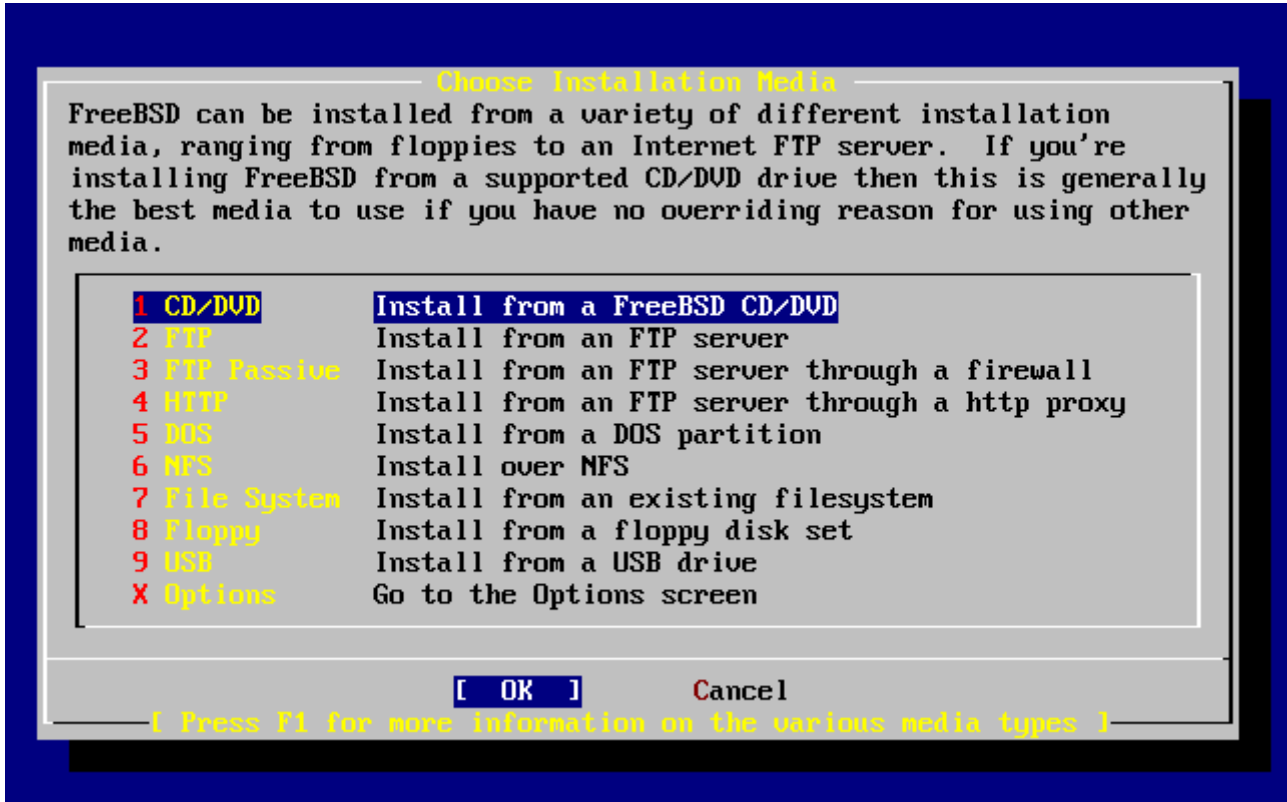
图 27. 安装介
