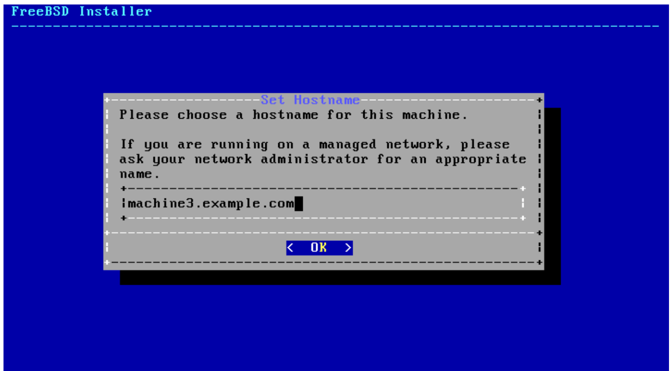
图 63. 设置主机名
